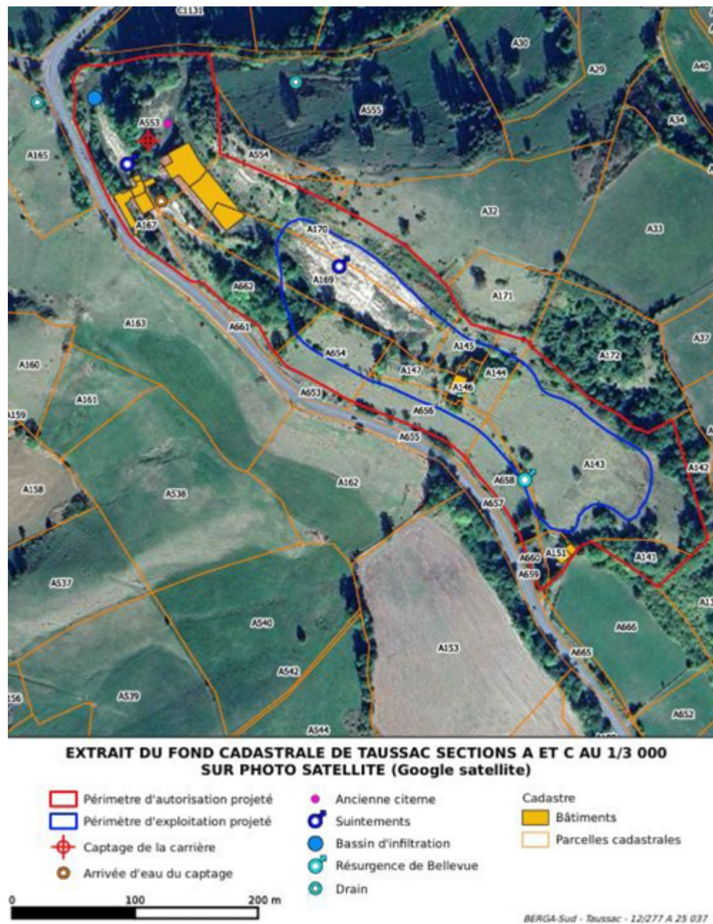
Figure I : situation cadastrale de la carrière et différents périmètres
