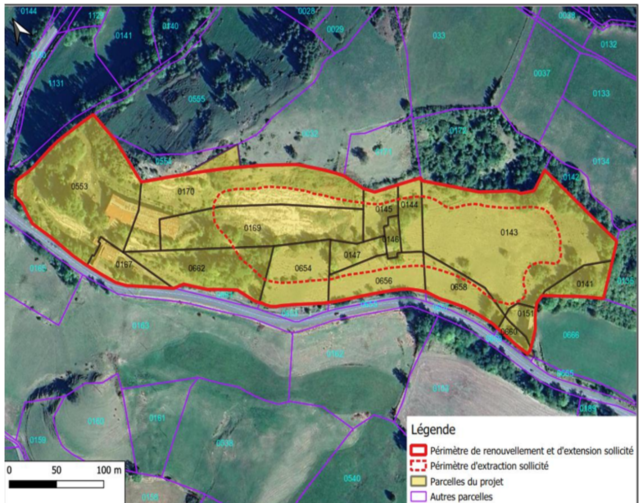
Figure 2 : Situation cadastrale de la carrière
